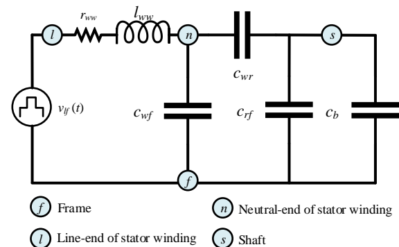
شکل (۲): مدار معادل مُد مشترک محرکه الکتریکی
