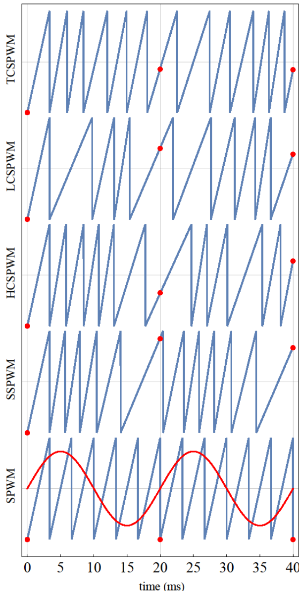
شکل (۶): سیگنالهای حامل در انواع مدولاسیون ( دامنه سیگنالهای حامل بین -۱ و +۱ همانند شکل ۵- هستند)
