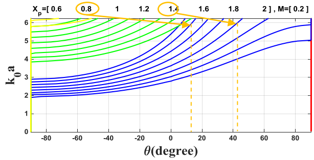
شکل (۲): نتیجه حل عددی معادله عمومی آنتن‌های موج نشتی و محاسبه زاویه تشعشع
