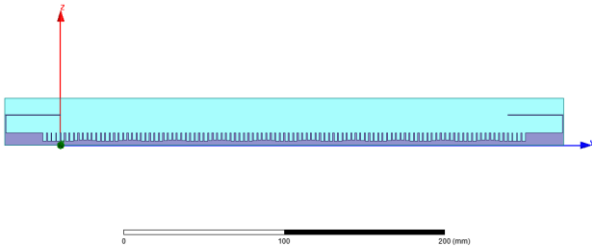
شکل (۵): ساختار نهایی آنتن موج نشتی دندان‌ایبا عمق متغیر
