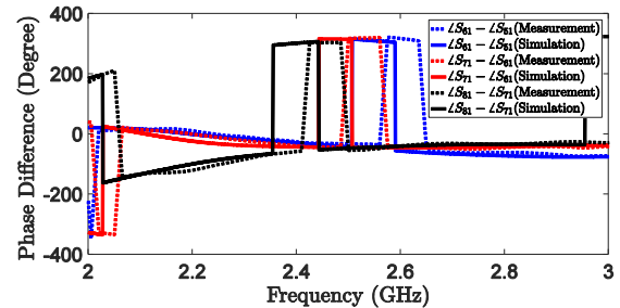
شکل (۲۲): نتایج اختلاف فازهای اندازه‌گیری شده ماتریس باتلر با تحریک دهانه اول
