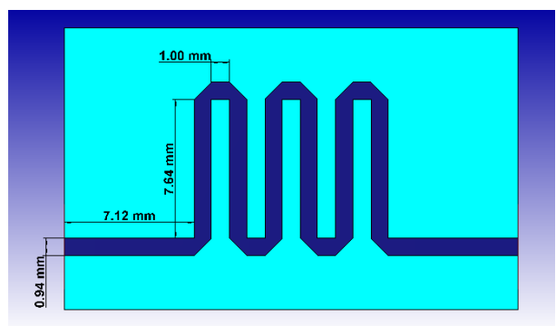
شکل (۱۲): تغییردهنده فاز شیفرن صفر درجه طراحی شده نتایج شبیه سازی در شکل های ۱۳ و ۱۴ آورده شده اند.
