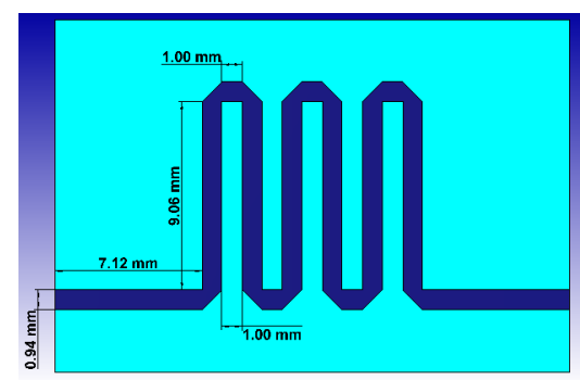
شکل (۹): تغییردهنده فاز شیفرن طراحی شده ۴۵- درجه
