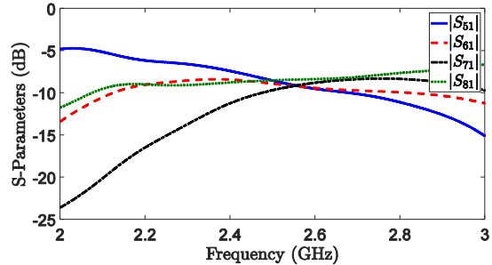
ب) پارامترهای پراکندگی سمت خروجی
