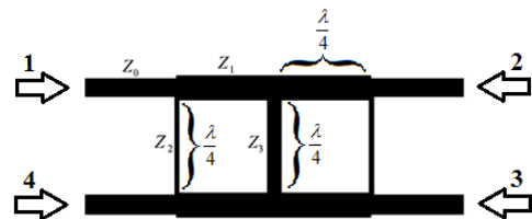
شکل (۲): تزویج کننده جهت‌دار شاخه‌ای دو بخشی پهن باند شده جدول (۲): امپدانس خطوط تزویج کننده ارایه شده در شکل ۲
