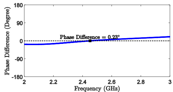
شکل (۱۴): نتیجه اختلاف فاز اشکال ارایه شده در شکل ۶ و ۱۲،
