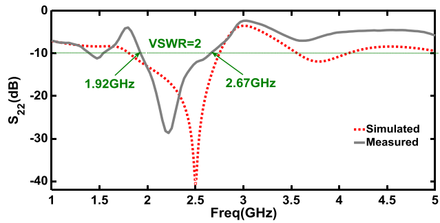
شکل (۶): منحنی شبیه سازی شده و اندازه گیری شده افت برگشتی برای پورت دو (S22)
