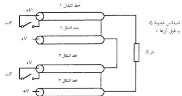
شکل (۱): ترسیم ساده ای از خط شکل دهی پالس BPFL دو حالتی
