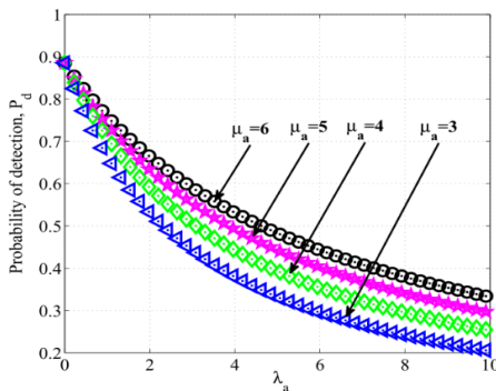
شکل (۷): احتمال آشکارسازی در مدل ترافیک مارکوف وابسته به زمان بر حسب \lambda_p و برای های متفاوت، برای L = 40 ، \lambda_a = \mu_a = 5 ، \gamma_p = \gamma_w = -1dB و T_s = 1ms ، \lambda = \mu = 5
