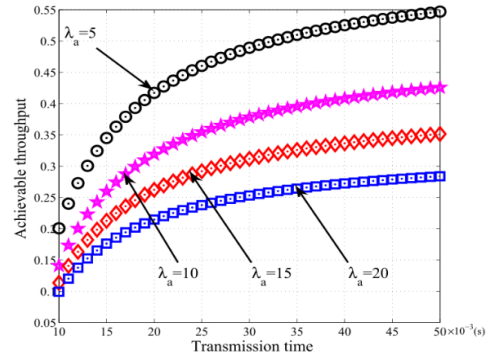
شکل (۸): برون‌دهی در دسترس برای شبکه کاربران ثانویه برحسب مدت‌زمان دوره انتقال و برای شدت ترافیک متفاوت و بر اساس \tau = 10ms, T_s = 1ms, J = 68, L = 40, \mu_p = \mu_a = \lambda = \mu = 5, \lambda_p = 30, \gamma_p = \gamma_w = 1(W) = 0dB و \gamma_s = -1dB
