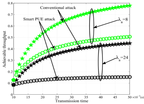
شکل (۱۰): مقایسه برون‌دهی برای شبکه کاربران ثانویه در حمله‌های سنتی و هوشمند، برحسب مدت‌زمان دوره انتقال و بر اساس \lambda_p = 30, \tau = 10ms, T_s = 1ms, J = 65, L = 50, \mu_a = 24, \mu_p = \lambda = \mu = 5
