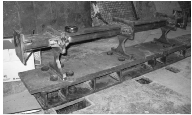
شکل ۵. تصویر یک نمونه آزمایشگاهی برشگیر فولادی.
