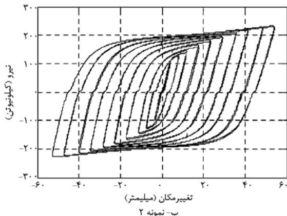
شکل ۱۱. منحنی رفتار نمونه‌های ۱ و ۲.
