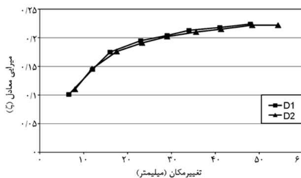
شکل ۱۳. میرایی ویسکوز معادل نمونه‌های ۱ و ۲.
