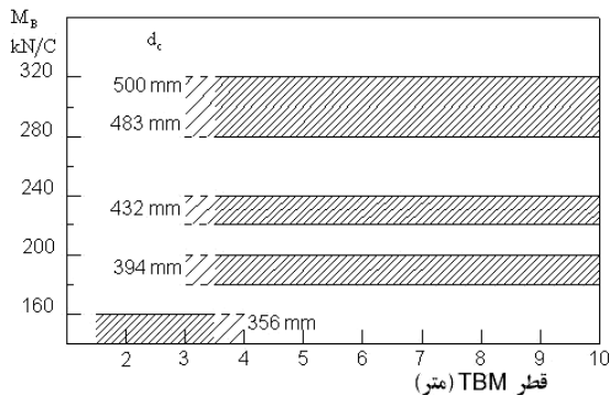
شکل ۳: میزان نیروی محوری اعمالی بر هر برش‌دهنده بر اساس قطر برش‌دهنده و تونل [۴]
