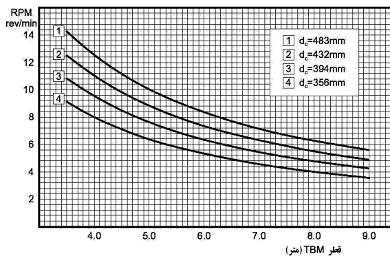
شکل ۴: رابطه سرعت چرخش پیشانی برشی با قطر ماشین و قطر برش‌دهنده [۴]
