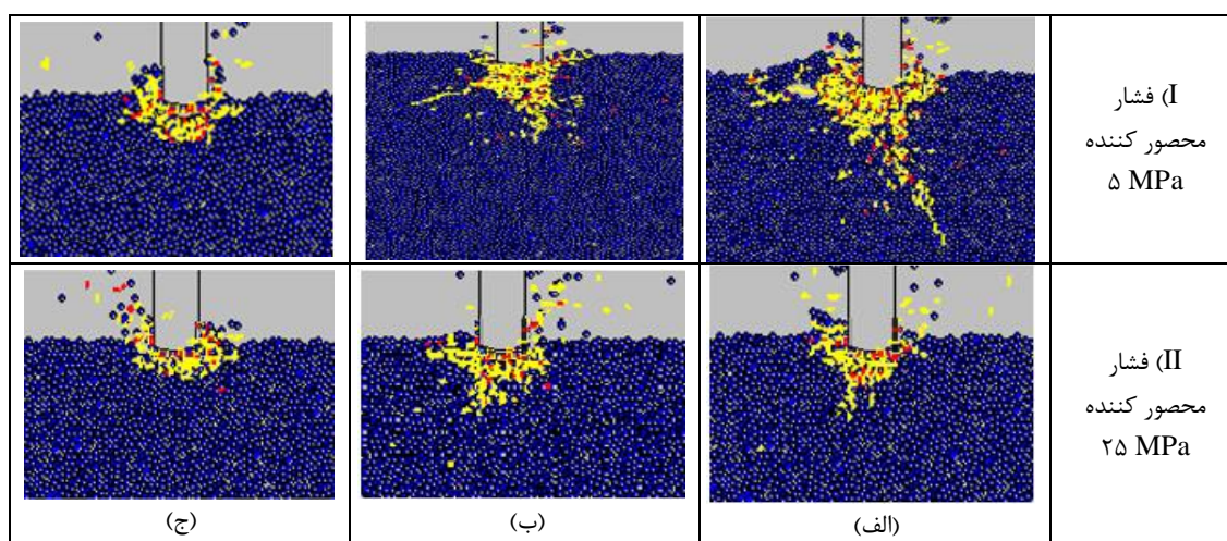
شکل ۹: توزیع شکست در مدل‌های با مقاومت کششی، الف) ۵ MPa، ب) ۱۰ MPa و ج) ۲۵ MPa
