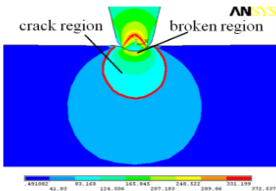
شکل ۱۳: ناحیه شکسته شده الاستیک و پلاستیک بیضوی زیر دیسک در نرم افزار ANSYS
