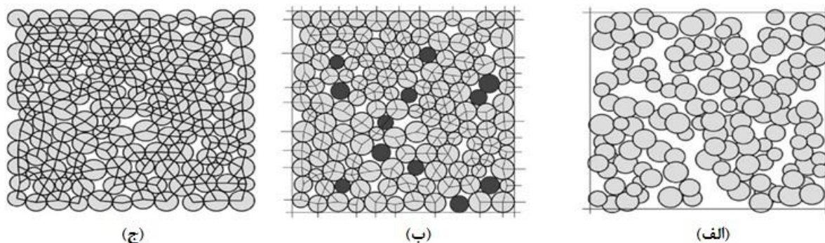
شکل ۳: نمایی از مراحل مختلف آماده‌سازی مدل، ایجاد مرزهای مدل و تولید دیسک‌ها، (ب) فشردگی اولیه ذرات، اعمال تنش ایزوتروپیک و کاهش تعداد ذرات معلق و (ه) اعمال پیوندهای موازی [۱۸]
