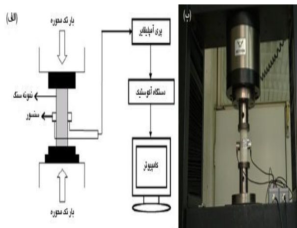
شکل ۵: دستگاه آکوستیک به همراه دستگاه بارگذاری
