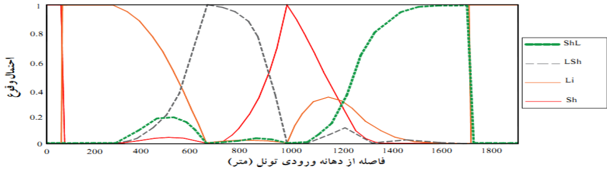
شکل ۱۲- نیمرخ پارامتر نوع سنگ بعد از به‌روزرسانی.
