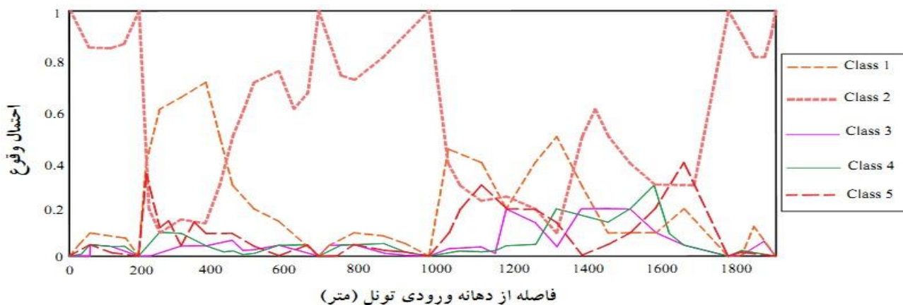
شکل ۹- نیمرخ کلاس زمین برای تونل گاران.
