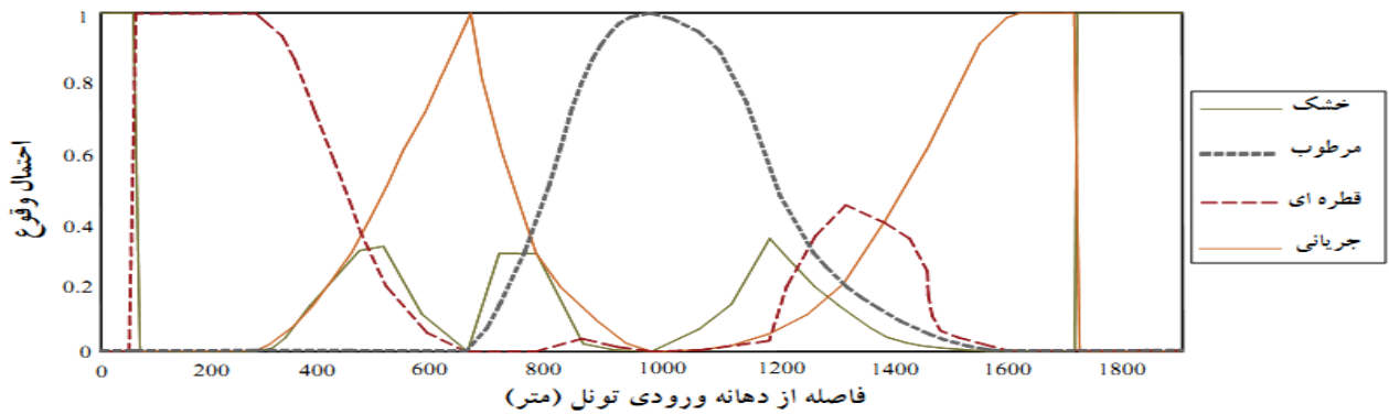
شکل ۱۴- نیمرخ پارامتر آب زیرزمینی بعد از به‌روزرسانی.
