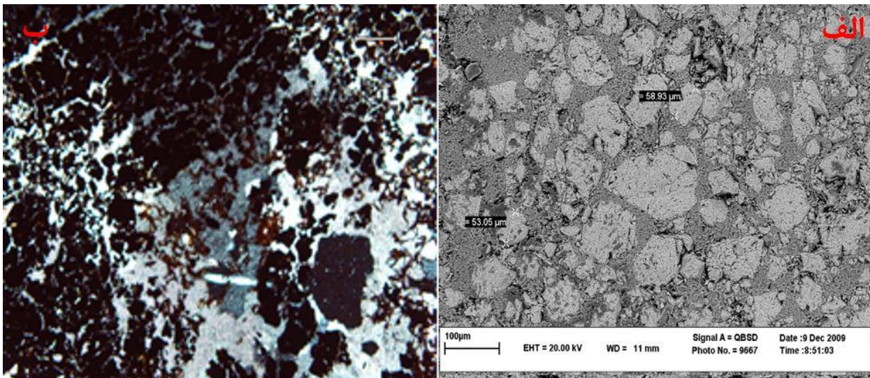
شکل ۵- الف) تصویر میکروسکوپ الکترونی از گرهک‌های هماتیتی که در آن دانه‌های هماتیت با سیمان کربناته به هم متصل شده‌اند، ب) تصویر میکروسکوپ نور عبوری، تبلور سیمان کربناته (رنگ روشن) در بین قطعات هماتیت (رنگ تیره) که به صورت سیمان آن‌ها را به یکدیگر چسبانده است.
