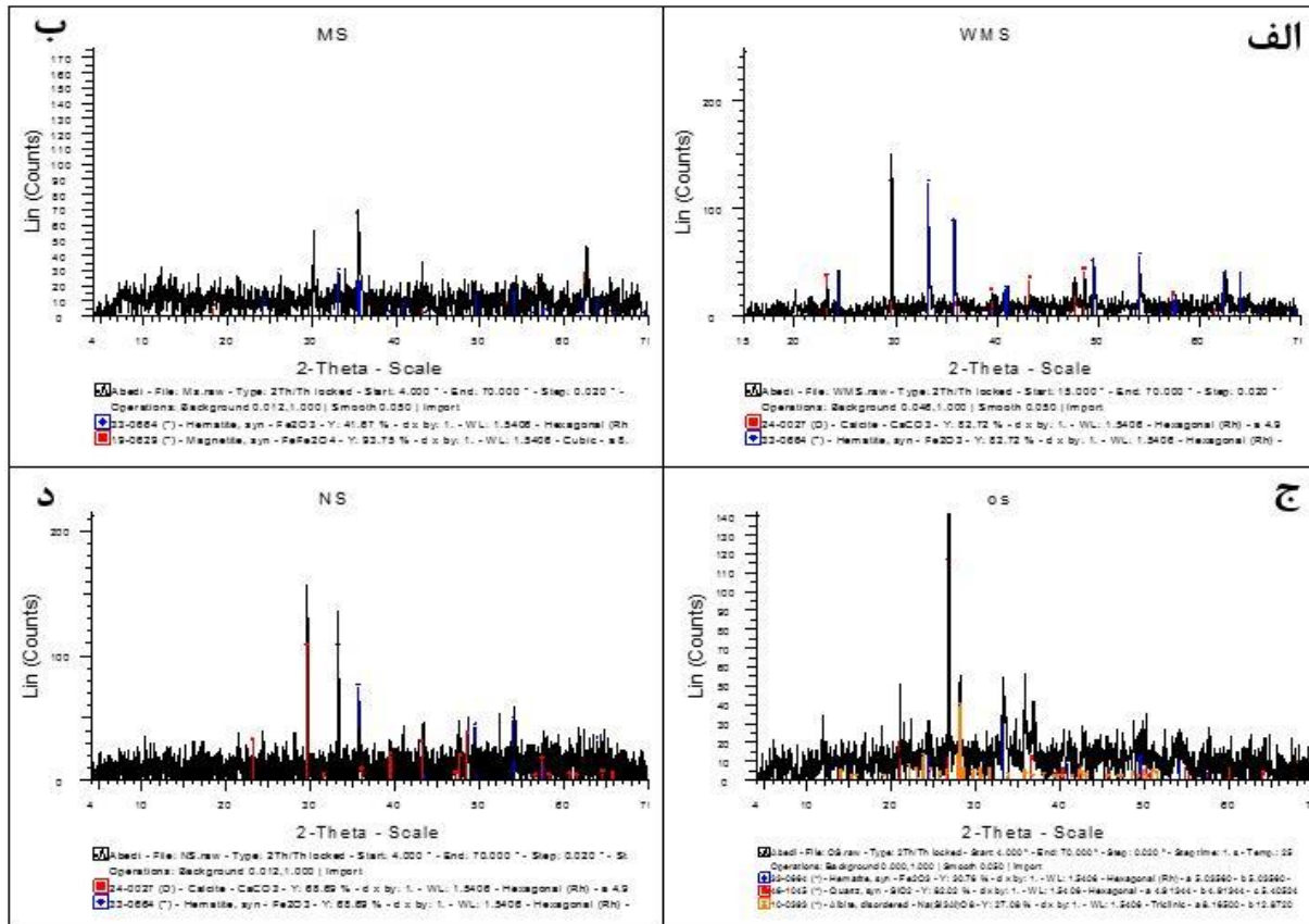
شکل ۴- نمودارهای پراش اشعه ایکس، (الف) نمونه سخت هماتیت، (ب) نمونه سخت هماتیت همراه با مگنتیت، (ج) نمونه آخری، (د) گرهک‌ها
