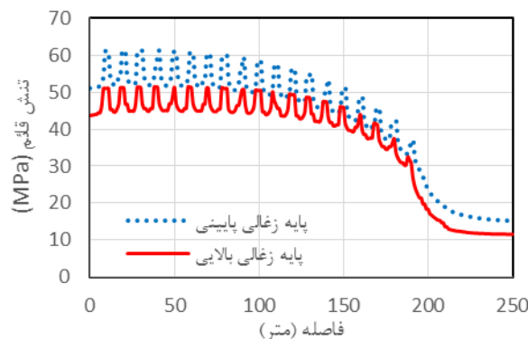
شکل ۲۰- تنش‌های قائم در پایه‌های زغال بالا و پایین (کارگاه و تونل‌ها برترتیب در موقعیت ۱۹۸ و ۲۱۰ متر)
