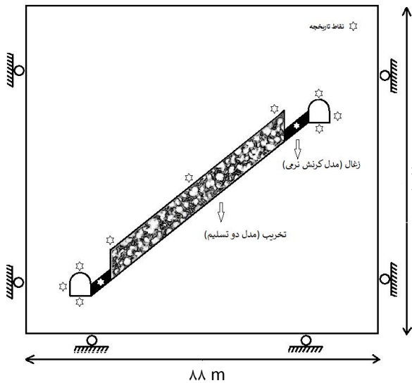
شکل ۲ نمای مدل عددی مورد استفاده در مطالعه حاضر
