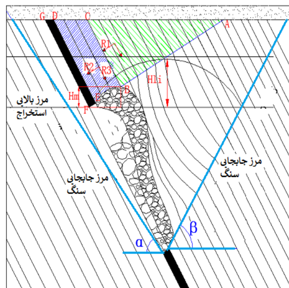
شکل ۱۶- تحلیل تنش‌ها در کارگاه جبهه کار بلند شیب دار (Xu et al., 2014)
