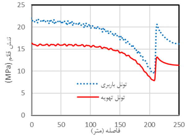
شکل ۱۲- تغییرات تنش‌های قائم در تاج تونل‌ها (کارگاه و تونل‌ها بترتیب در موقعیت ۱۹۸ و ۲۱۰ متری)
