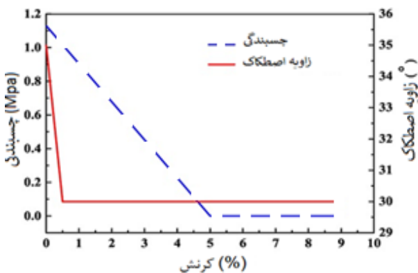
شکل ۴- تغییرات چسبندگی و اصطکاک با کرنش پلاستیک اعمال شده در مطالعه حاضر (Zhao et al, 2014)
