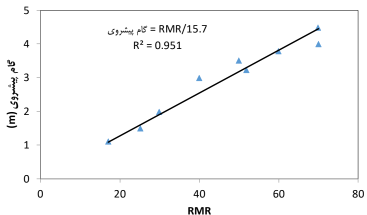
شکل ۴ - (الف) طول گام پیشروی بر حسب RMR برای قسمت طاق تونل. (ب) طول گام پیشروی بر حسب RMR برای قسمت پاتاق تونل در شرایط چال‌های افقی
