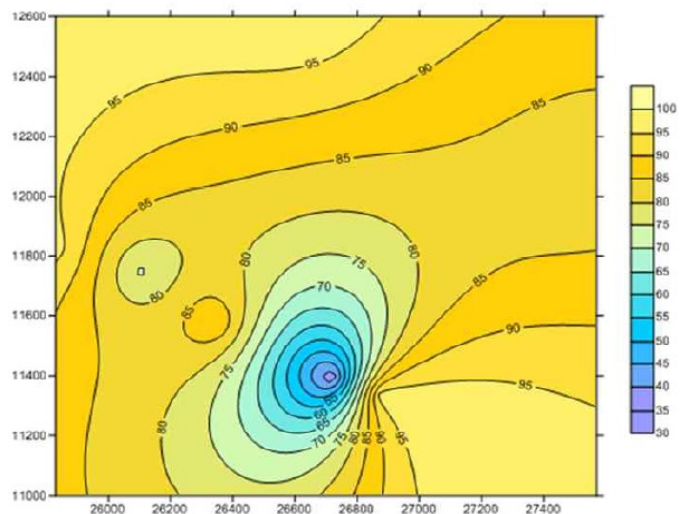
شکل ۲ - نمونه‌ای از نتایج مدل‌سازی ویژگی‌های زمین‌شناسی با استفاده از اطلاعات گمان‌های در یک سطح تراز مشخص به کمک نرم‌افزار Surfer
