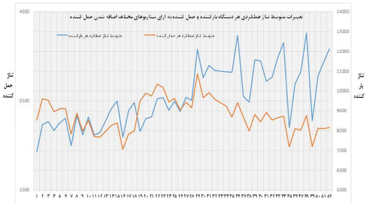
شکل ۶: مقایسه تغییرات متوسط تناژ عملکرد بارکننده و حمل کننده در هر یک از سناریوهای افزایش حمل کننده‌ها.
