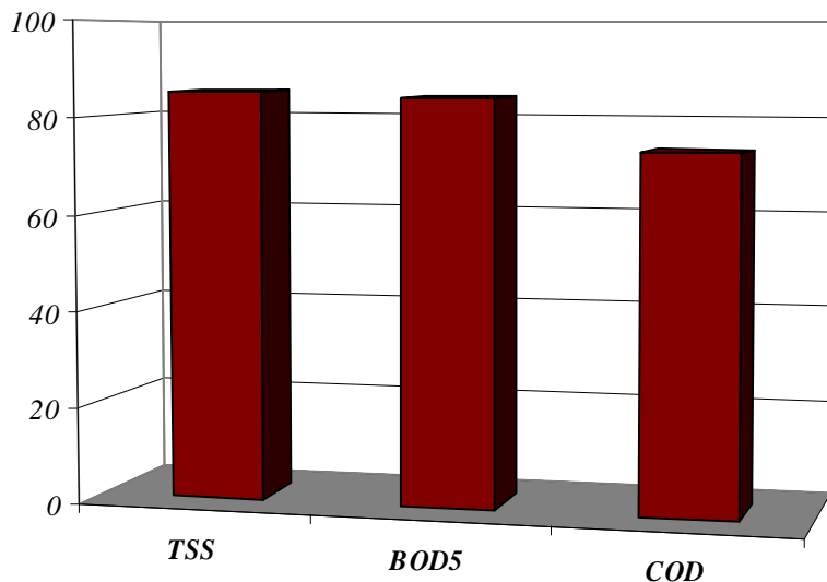
نمودار 1. درصد حذف مولفه های آلاینده مورد توجه در فاضلاب با سیستم لجن فعال به روش هوادهی ریزشی
