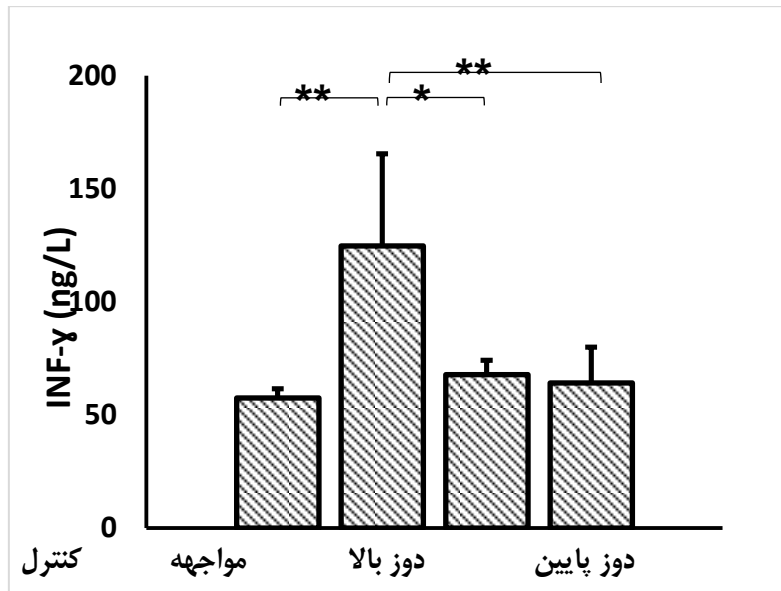
نمودار شماره ۱. اثر 5-HMF در دوز ۱۸۸ و ۷۵۰ (mg/kg bw) بر سطوح سرمی IL-4 و IFN-γ در موش های BALB/c ایمونیزه شده با اوآلبومین. هر ستون mean±S.E.M را نشان می دهد. *P<0.05، **P<0.01، ***P<0.001.
