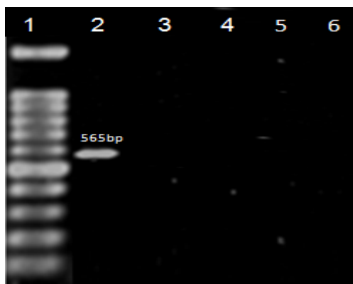
شکل شماره ۳. ژل آگاروز مربوط به اختصاصیت واکنش PCR با استفاده از باکتری های مختلف ستون ۱ (نشانگر اندازه DNA (100 bp DNA Ladder)، ستون ۲ سویه ETEC، ستون ۳ کلبسیلا پنومونیه، ستون ۴ سودوموناس آنروژینوزا، ستون ۵ سالمونلاتیفی، ستون ۶ شیگلا دیسانتریه
