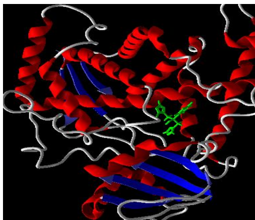
شکل شماره ۱. داکینگ مولکول فلوکونازول (سبز رنگ) در جایگاه فعال آنزیم لانسترول ۱۴ آلفا دمیتلاز
