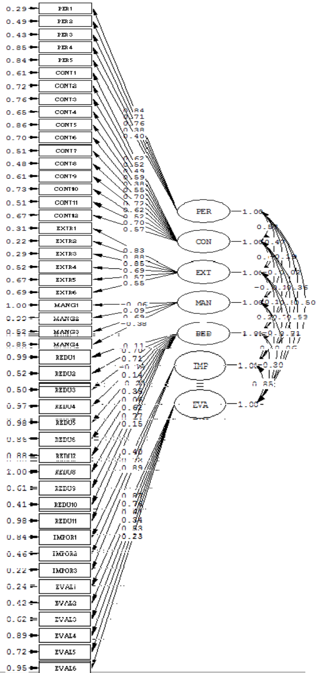
شکل ۱: نتایج تحلیل عاملی در حالت تخمین استاندارد
