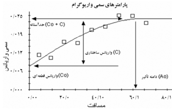
شکل ۱: سمی واریوگرام ایده‌آل همراه با پارامترهای مربوطه
