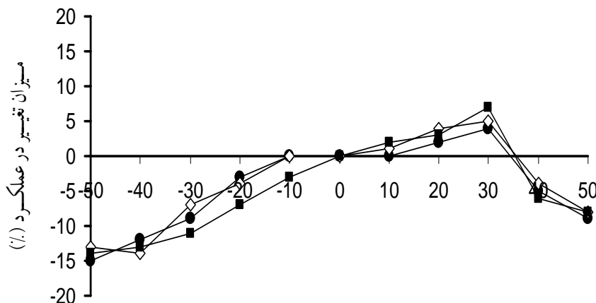
شکل ۲- حساسیت عملکرد شبیه سازی شده گندم به تغییرات تراکم کاشت در محدوده \pm 50 درصد نسبت به مقدار مینا (۴۰۰ بوته در متر مربع) در سه استان خراسان
