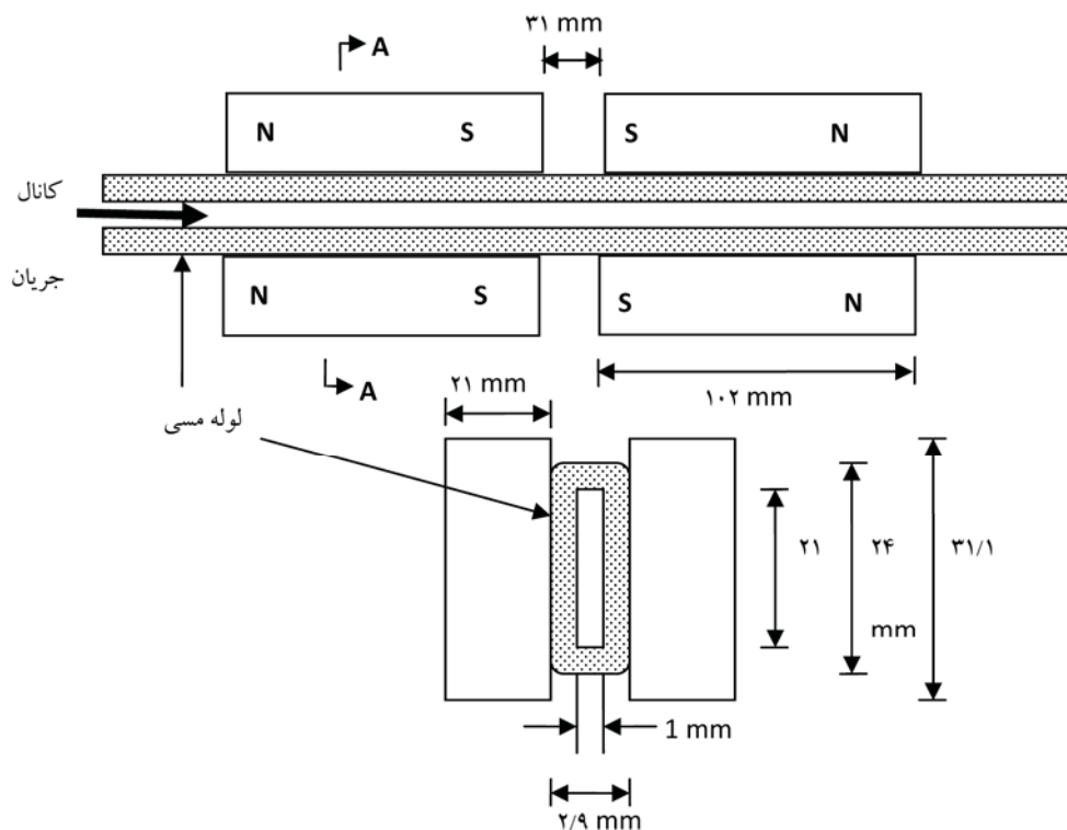
شکل ۱- آرایش میدان مغناطیسی دائمی و اندازه کانال عبور محلول و قطعات آهن رباها
