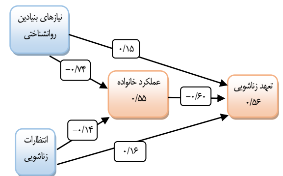
شکل ۲. مدل نهایی مسیرهای آزمون شده به همراه آماره‌های پیش‌بینی استاندارد شده توجه: اعداد روی خطوط مسیر و داخل مستطیل‌ها به ترتیب، ضرایب بتا و ضرایب تبیین هستند.
