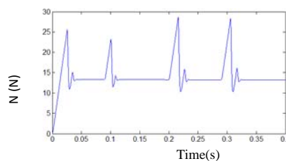
شکل (۱۴) نیروی عمود بر سطح در مانور ترکیبی جسم توسط میج و انگشتان
