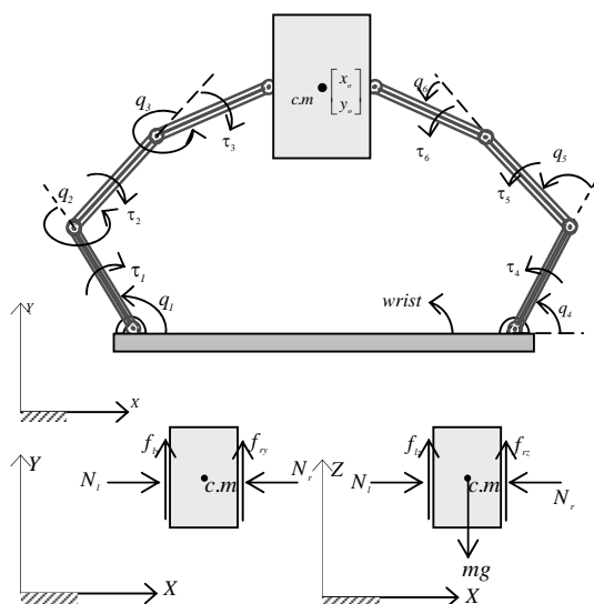
شکل (1) شماتیک سیستم مورد مطالعه و دیاگرام آزاد جسم گرفته شده
