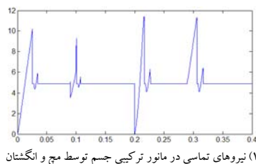
شکل (۱۵) نیروهای تماسی در مانور ترکیبی جسم توسط میج و انگشتان
