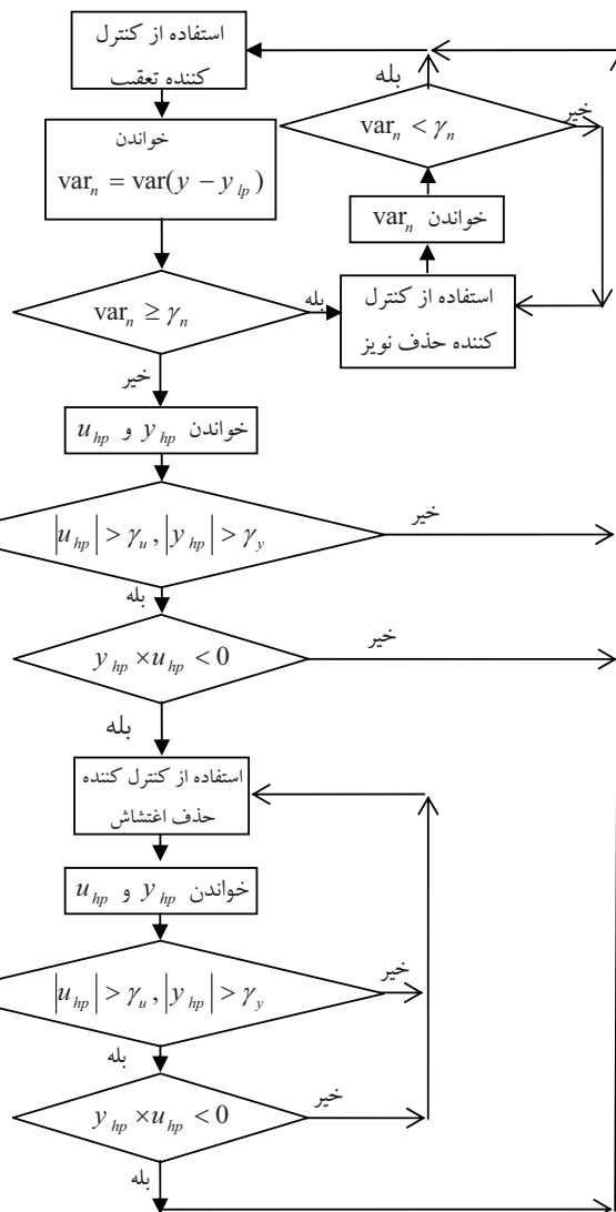
شکل ۶: الگوریتم انتخاب کنترل کننده توسط سرپرست
