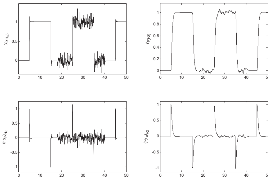
شکل ۷: به ترتیب از سمت راست، پاسخ حلقه بسته کنترل کننده های K_{H_2} و K_{H_\infty} منحنی بالا خروجی y_p و منحنی های پایین خطای تعقیب y_p - r مثال ۱
