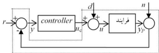
شکل ۲: پیکربندی حلقه بسته
