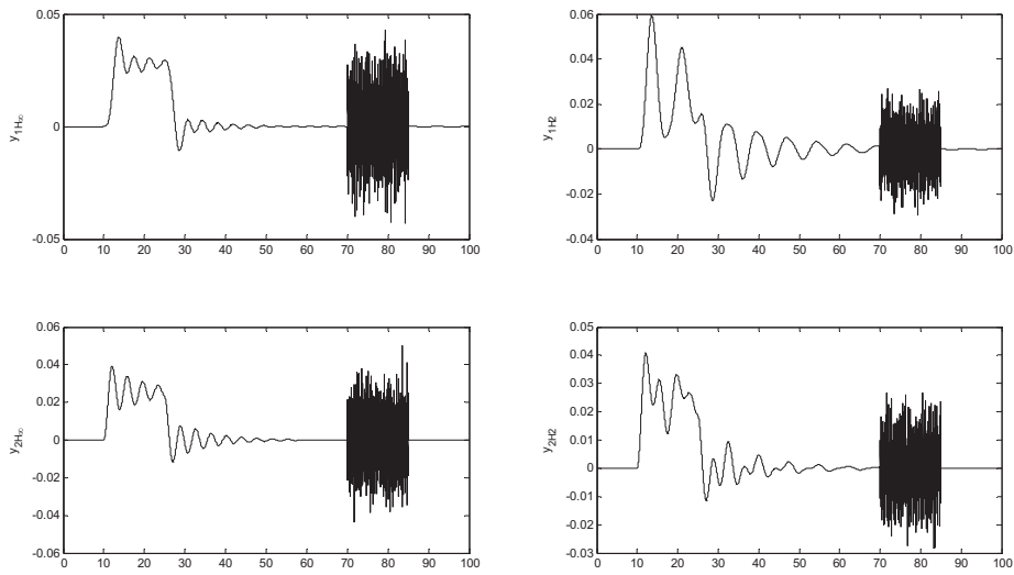
شکل ۱۰: پاسخ حلقه بسته کنترل کننده‌های K_{H_2} و K_{H_1} مثال ۲
