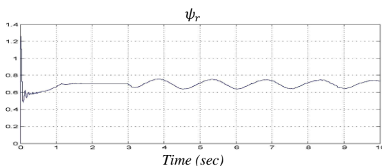
شکل ۱۰: عملکرد موتور فقط با وجود کنترل‌کننده نامی در حضور خطای مکانیکی رتور
