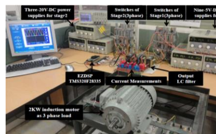
شکل ۸: نمونه آزمایشگاهی پیاده‌سازی شده از مبدل ۱۶ سطحی سه فازه بر اساس آنچه در شکل ۷ نشان داده شده است
