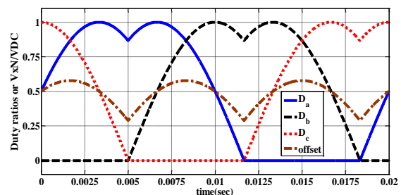
شکل ۶: نسبت‌های وظیفه سه فازه محاسبه شده در تکنیک مدولاسیون افست
