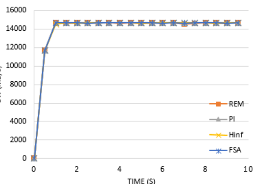
شکل ۱۵: نمودار حذف بسته و پهنای باند لینک گلوگاه مسیریاب در آزمایش ششم
