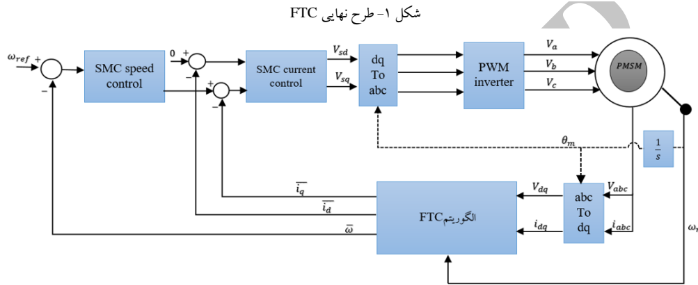
شکل ۲- بلوک دیاگرام کلی طرح FTC پیشنهادی
