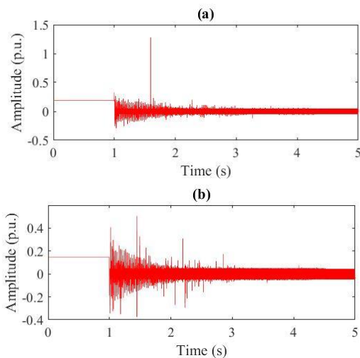
شکل ۳: نمودارهای (a) و (b) به ترتیب مربوط به سیگنال‌های ولتاژ روتور در راستای محور d v_{dr}(t) و محور q v_{qr}(t) ورودی‌های کنترل حاصل شده به روش SDRE
