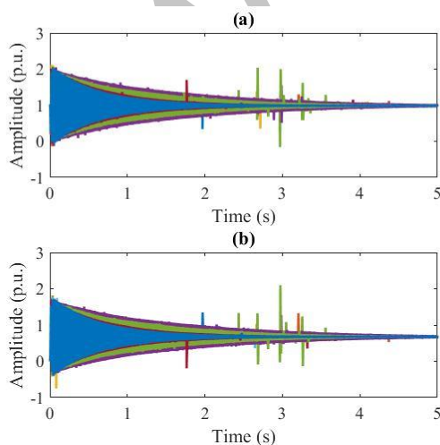
شکل ۴: نمودارهای (a) و (b) به ترتیب مربوط به سیگنال‌های جریان استاتور در راستای محور d i_{ds}(t) و محور q i_{qs}(t) ، با وجود نامعینی در پارامترها.
