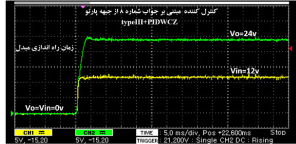
شکل (۱۲) - پاسخ عملی میدل بوست در شرایط راه اندازی مربوط به کنترل کننده کلاسیک typeIII و کنترل کننده بهینه مبتنی بر جواب شماره ۸ از جبهه پارتو typeIII+PIDW CZ
