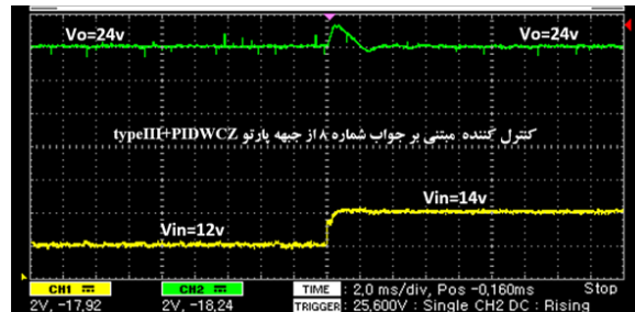
شکل (۱۵) - پاسخ عملی میدل بوست در شرایط تغییر ولتاژ ورودی مربوط به کنترل کننده کلاسیک typeIII و کنترل کننده بهینه مبتنی بر جواب شماره ۸ از جبهه پارتو typeIII+PIDW CZ
