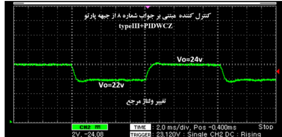
شکل (۱۴) - پاسخ عملی میدل بوست در شرایط تغییر ولتاژ مرجع مربوط به کنترل کننده کلاسیک typeIII و کنترل کننده بهینه مبتنی بر جواب شماره ۸ از جبهه پارتو typeIII+PIDW CZ
