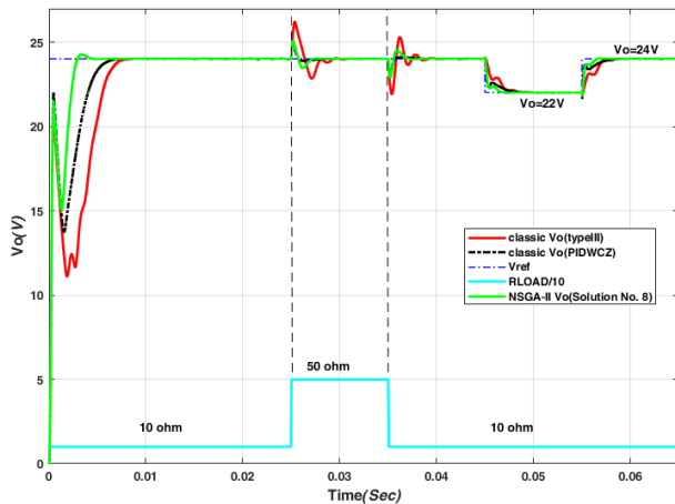
شکل (۷) - پاسخ حاصل از کنترل کننده های کلاسیک و کنترل کننده بهینه پیشنهادی بر اساس جواب شماره ۸
