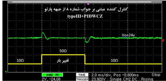
شکل (۱۳) - پاسخ عملی میدل بوست در شرایط تغییر بار مربوط به کنترل کننده کلاسیک typeIII و کنترل کننده بهینه مبتنی بر جواب شماره ۸ از جبهه پارتو typeIII+PIDW CZ
