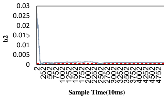
شکل ۱۳ همگرایی پارامترهای مدل آنلاین به آفلاین تابع تبدیل سرعت به جریان
