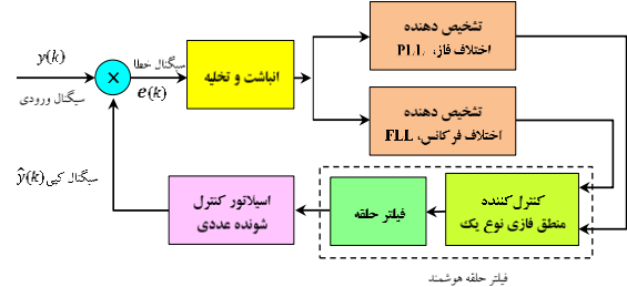
شکل ۵: حلقه قفل شونده فاز با استفاده از منطق فازی نوع اول [۱۳].
