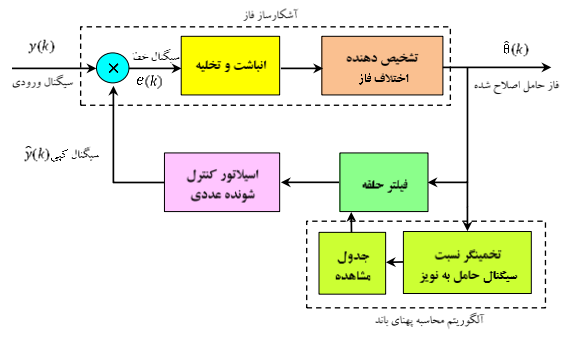
شکل ۴: حلقه قفل شونده فاز با پهنای باند از قبل محاسبه شده [۱۲] ۴-۲-۳ حلقه قفل شونده فاز با استفاده از منطق فازی نوع اول
