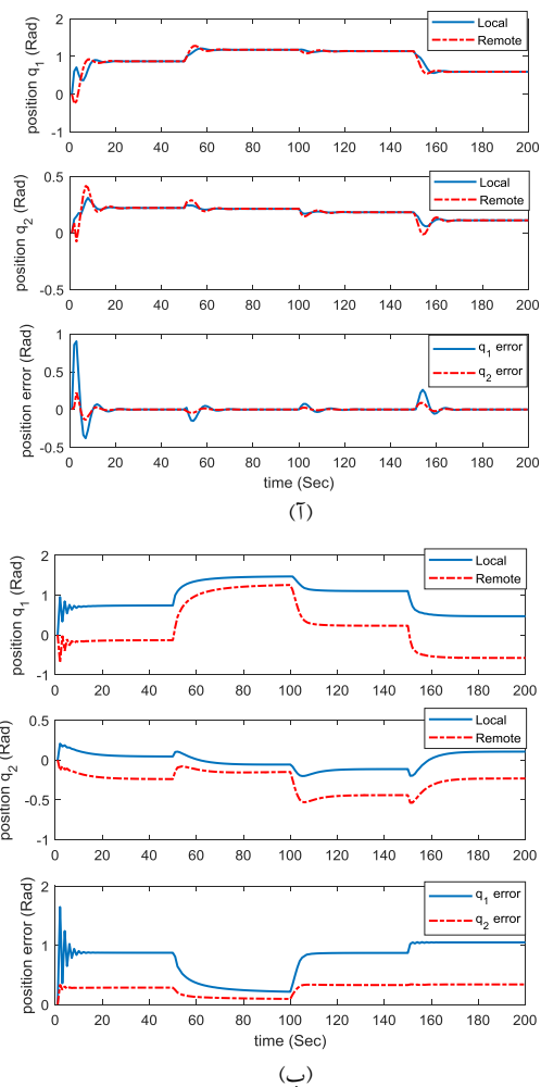
شکل ۶: موقعیت و خطای ردیابی موقعیت در سیستم عمل از دور کنترل شونده با (آ) با روش موردنظر (ب) با روش مقاله [۲۰] در فضای مفصلی.
