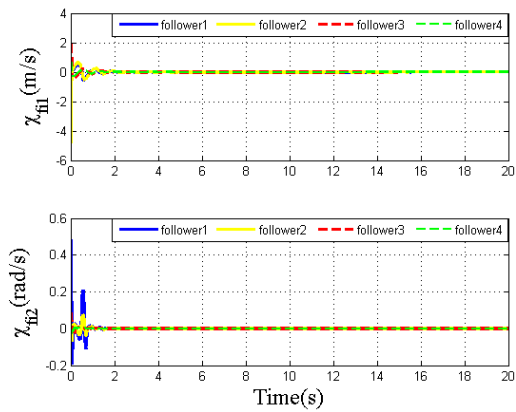
شکل ۱۷: خطای خروجی فیلترها
