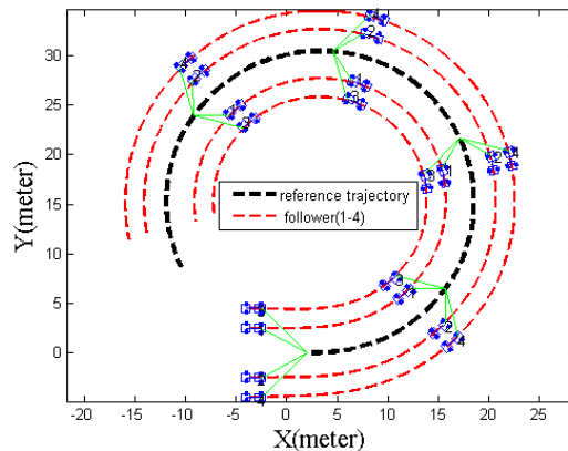
شکل ۹: ردیابی مسیر زمانی مرجع توسط ربات های پیرو
