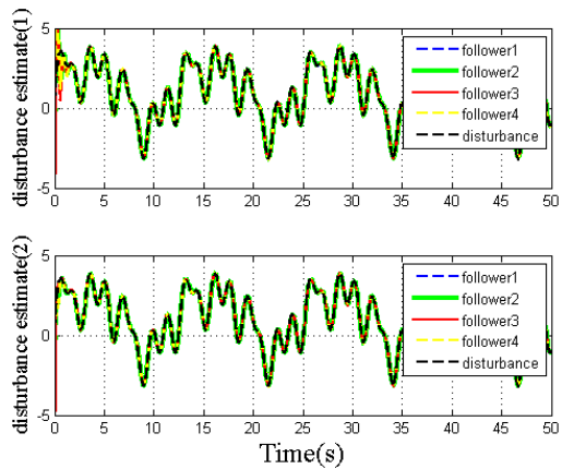
شکل ۷: تخمین اغتشاشات خارجی
