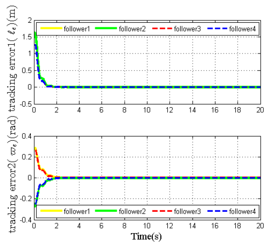
شکل ۴: خطای ردیابی موقعیت و جهت گیری
