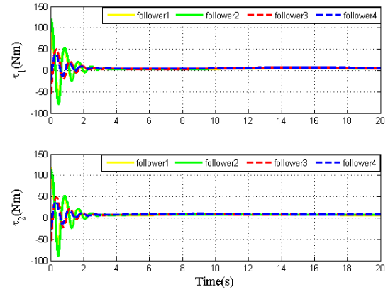
شکل ۱۶: گشتاورهای ورودی
