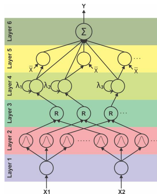
شکل 8: ساختار RSEFNN
