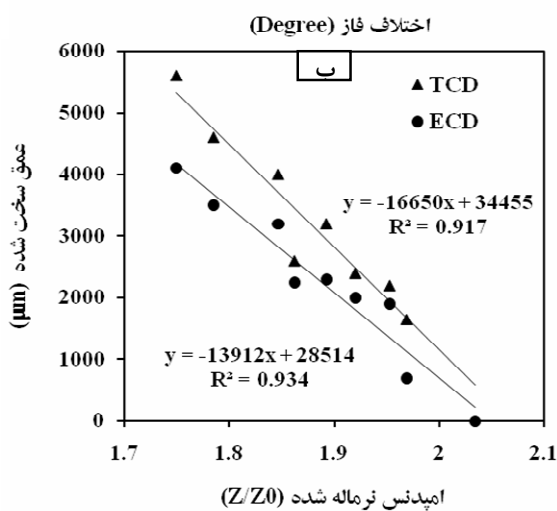
شکل ۷. ارتباط بین عمق لایه سخت شده کل و مؤثر (الف) اختلاف فاز ولتاژ و جریان (ب) امپدانس نرماله شده، در فرکانس ۲۵ هرتز.
