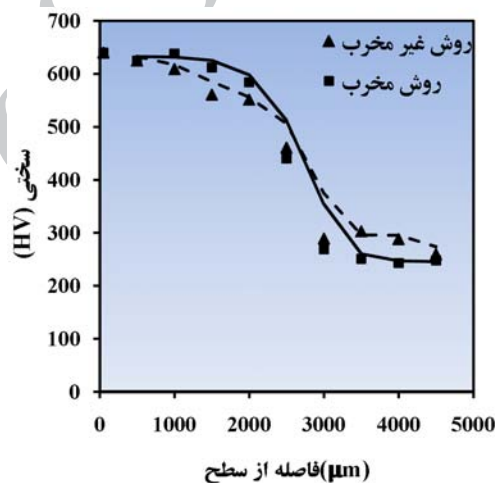
شکل ۱۱. پروفیل های سختی با استفاده از دو روش مخرب و غیر مخرب.
