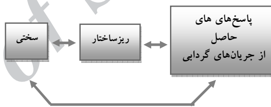
شکل ۹. نمودار شماتیک تأثیر سختی و ریزساختار بر پاسخ های حاصل از جریان های گردابی.
