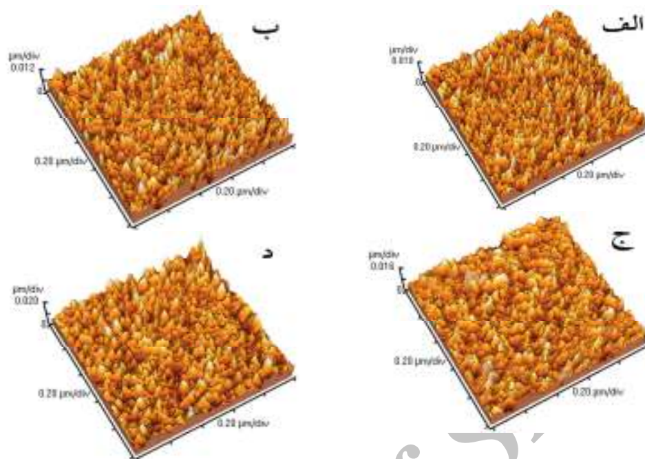
شکل ۵. تصاویر AFM (سه بعدی) سطح لایه های نازک تیتانیم ایجاد شده در مدت زمان های الف (۵ min، ب) ۱۰ min، ج) ۱۵ min و د) ۲۰ min
