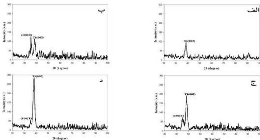
شکل ۷. الگوهای XRD لایه های نازک تیتانیم ایجاد شده در مدت زمان های الف) ۵ min، ب) ۱۰ min، ج) ۱۵ min و د) ۲۰ min
