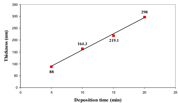
شکل ۱. منحنی تغییرات ضخامت لایه های نازک تیتانیوم نسبت به مدت زمان رسوب دهی
