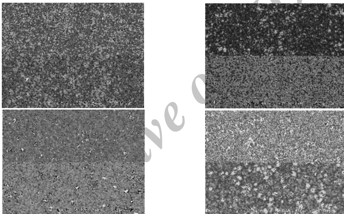
شکل ۳. تصاویر FESEM سطح لایه های نازک تیتانیم ایجاد شده در مدت زمان های الف) ۵ min، ب) ۱۰ min، ج) ۱۵ min و د) ۲۰ min
