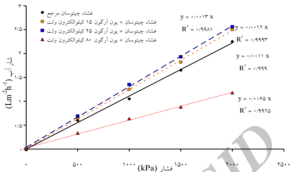
شکل ۵. منحنی شار آب عبوری از غشاء چیتوسان مرجع و نمونه‌های پردازش شده با باریکه یونی آرگون با انرژی‌های ۱۵، ۲۵ و ۸۰ کیلو الکترون ولت و با شار 5 \times 10^{15} \text{ ion/cm}^2 بر حسب افزایش فشار
