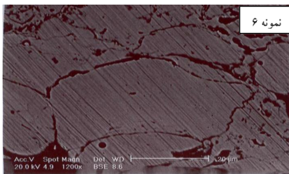
شکل ۳. تصاویر بدست آمده توسط SEM سطح مقطع شش نمونه قبل از خوردگی با بزرگنمایی بالاتر
