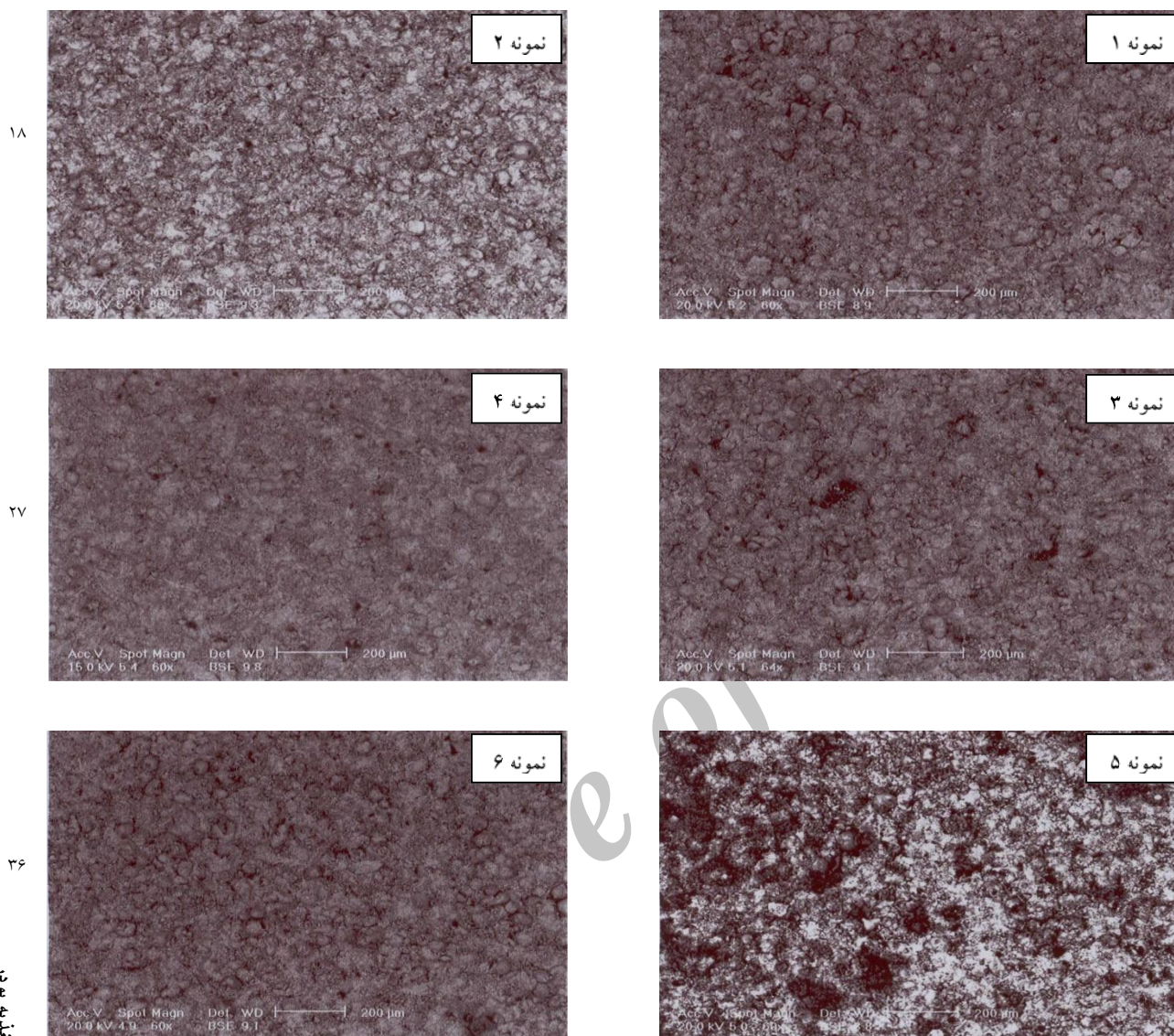
نسبت سوخت به اکسیژن نمونه های ۲، ۴ و ۶ = ۱/۲۵
