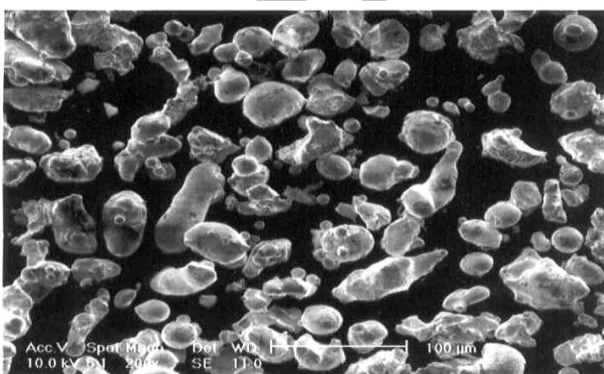
شکل ۱. شکل و اندازه ذرات پودر اولیه نیکل کروم
