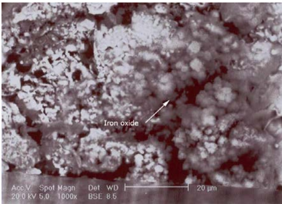
شکل ۷: تصویر بدست آمده توسط SEM نمونه شماره ۵ با بزرگنمایی بالاتر بعد از خوردگی
