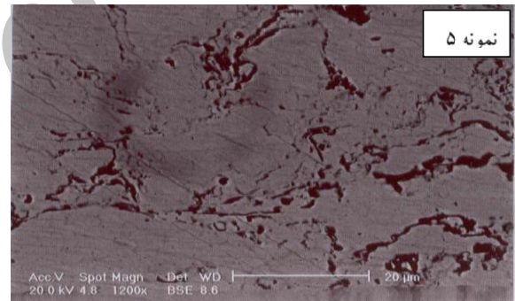
شکل ۳. تصاویر بدست آمده توسط SEM سطح مقطع شش نمونه قبل از خوردگی با بزرگنمایی بالاتر
