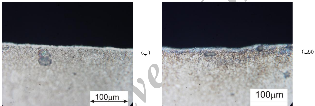
شکل ۷. تصویر میکروسکوپ نوری با بزرگنمایی ۵۰۰X (الف) سیکل وظیفه ۲۰٪ (ب) سیکل وظیفه ۳۰٪ (زمان روشنی پالس: ۲ میکروتانیه و قطبیت منفی)
