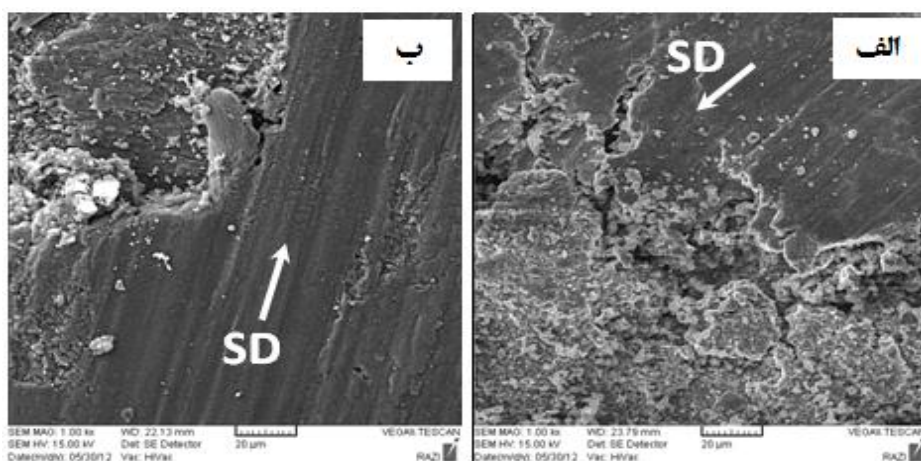
شکل ۸. تصویر میکروسکوپی الکترونی از سطح سایش (SD: جهت لغزش) آلیاژ \text{Al-5Si} (الف) و آلیاژ \text{Al-13Si} (ب)
