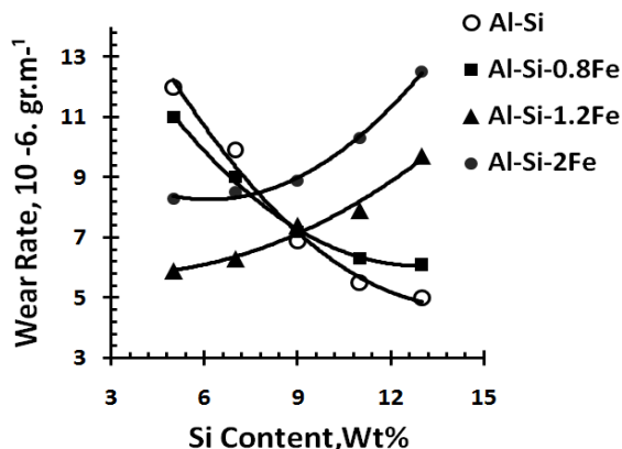
شکل ۲. تغییرات نرخ سایش بر حسب میزان سیلیسیم برای آلیاژهای دوتایی \text{Al-Si} حاوی مقادیر مختلف آهن.
