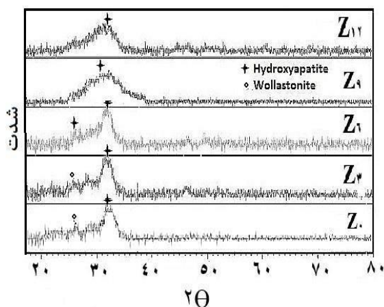
شکل ۱. الگوی پراش اشعه ایکس نمونه شیشه - سرامیک کلسیم فسفاتی و نمونه های حاوی ۰، ۳، ۶، ۹ و ۱۲ درصد زیرکونیا.
