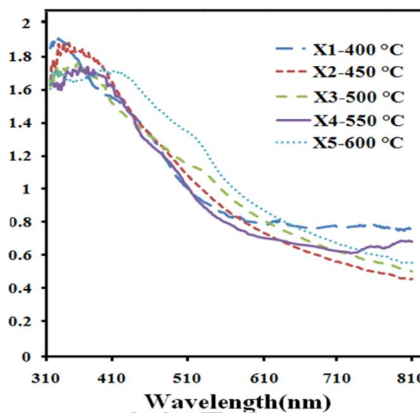
شکل ۵. نمودار طیف جذبی لایه نازک مگه‌مایت ( \gamma\text{-Fe}_2\text{O}_3 ) برای تمام دماهای باز پخت
