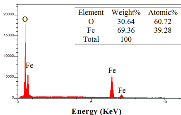
شکل ۸. تصویر EDX از نمونه مربوط به نانوذره باز پخت نشده
