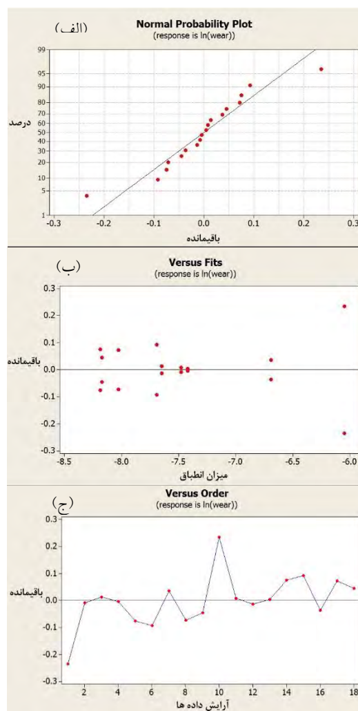
شکل ۱۴. نمودارهای الف) احتمال نرمال بودن، ب) میزان پراکندگی و ج) میزان مستقل بودن داده‌ها
