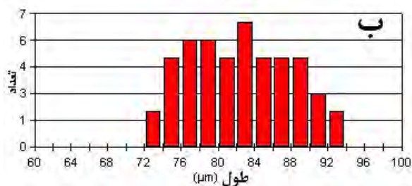
شکل ۹. نمودار توزیع ضخامت پوشش در سطح مقطع نمونه‌های الف (شماره ۱ و ب) شماره ۵
