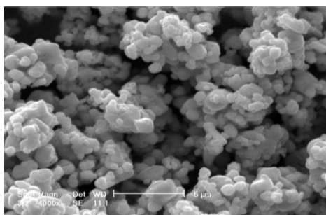
شکل ۱. پودر نقره با اندازه دانه متوسط ۰/۵ میکرون
