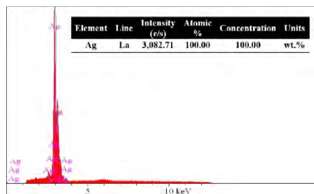
شکل ۲. درصد میزان خلوص نقره به کمک آزمون EDS
