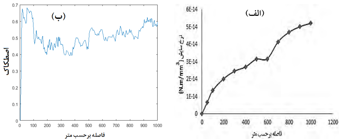
شکل ۱۳. نمودارهای الف) نرخ سایش و ب) ضریب اصطكاك بر حسب مسافت سایش مربوط به نمونه بهینه
