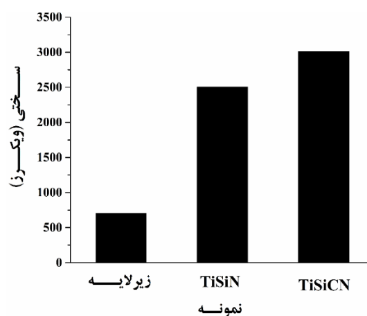
شکل ۳. سختی پوشش‌های TiSiCN ، TiSiN و زیرلایه
