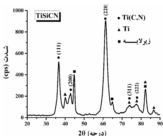
شکل ۱. الگوی پراش پرتو ایکس پوشش TiSiCN
