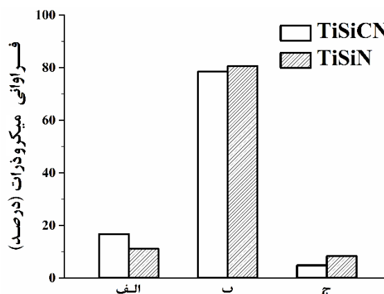
شکل ۸. نمودار درصد مشارکت هر گروه از میکروذرات در پوشش‌های TiSiN و TiSiCN .
