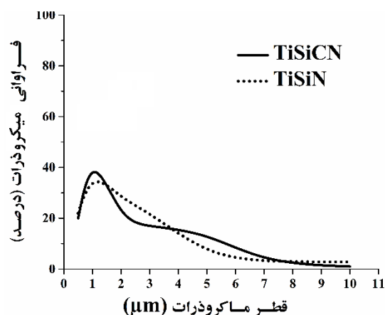
شکل ۷. توزیع کلی میکروذرات برحسب قطر در پوشش‌های TiSiN و TiSiCN .
