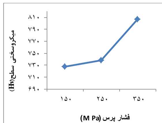
شکل ۹. تأثیر فشار پرس بر سختی سطح قطعه کار لایه نشانی شده با تخلیه الکتریکی: ترکیب الکترود: شماره ۲، سیکل وظیفه=۲۰٪.
