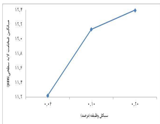
شکل ۸. تأثیر سیکل وظیفه بر ضخامت لایه سطحی لایه نشانی شده با تخلیه الکتریکی. V=200v ، ترکیب الکتروود: شماره ۳، P=250Mpa
