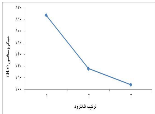
شکل ۱۰. تاثیر ترکیب شیمیایی الکترود بر سختی سطح قطعه کار V=200v, P=350Mpa
