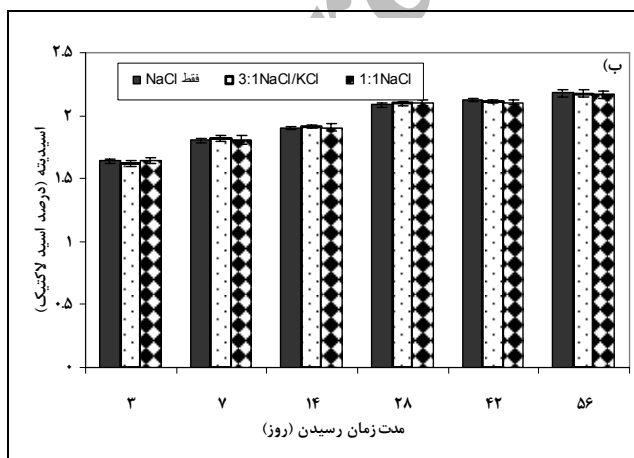
شکل ۱ - (الف) تغییرات pH و (ب) تغییرات اسیدیته در نمونه‌های پنیر رسیده در محلول‌های ۱۰٪ نمک طعام و نسبت‌های مختلف
