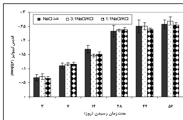
شکل ۷ - تغییرات اندیس لیپولیز در نمونه‌های پنیر رسیده در آب نمک ۰/۱۰ حاوی NaCl یا نسبت‌های متفاوت NaCl/KCl طی دوره رسیدن
