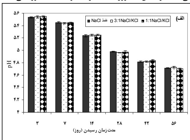
شکل ۱ - (الف) تغییرات pH و (ب) تغییرات اسیدیته در نمونه‌های پنیر رسیده در محلول‌های ۱۰٪ نمک طعام و نسبت‌های مختلف
