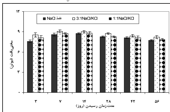
شکل ۸ - تغییرات بافت در نمونه‌های پنیر رسیده در آب نمک ۰/۱۰ حاوی NaCl یا نسبت‌های متفاوت NaCl/KCl طی دوره رسیدن
