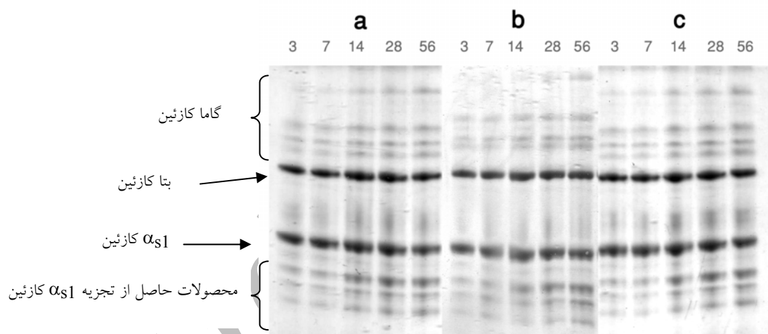
شکل ۶ - الکتروفوروگرام مربوط به نمونه‌های پنیر تهیه شده در آب نمک ۰/۱۰ حاوی نسبت‌های متفاوت NaCl/KCl طی دوره رسیدن: (a) نمونه پنیر رسیده در آب نمک حاوی نسبت‌های ۳:۱ NaCl/KCl، (b) ۱:۱ NaCl/KCl و (c) NaCl به تنهایی
