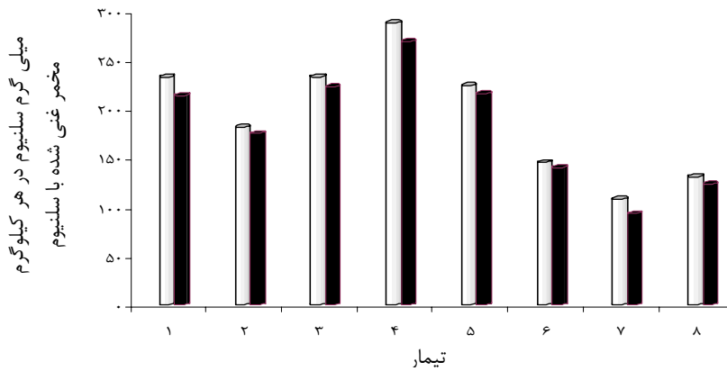
نمودار ۱. مقایسه بازده نهایی بیوترانسفورماسیون سلینیوم (نمودار سفید رنگ) و مقدار سلینیوم آلی تجمع یافته در سلول‌های مخمیری (نمودار مشکی رنگ) طی آزمون‌های مختلف انجام شده طبق طرح پلاکت برمن
